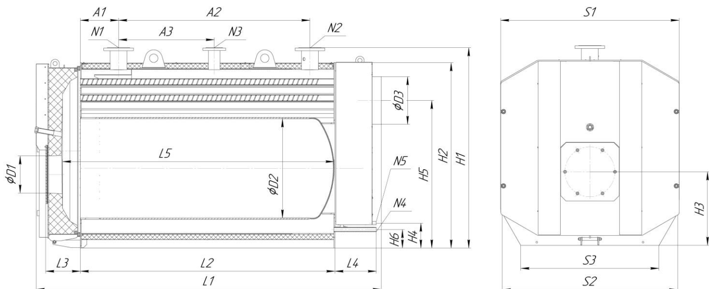
Рисунок 1. Внешний вид котлов Titan Prom 2000 - 4000 кВт
